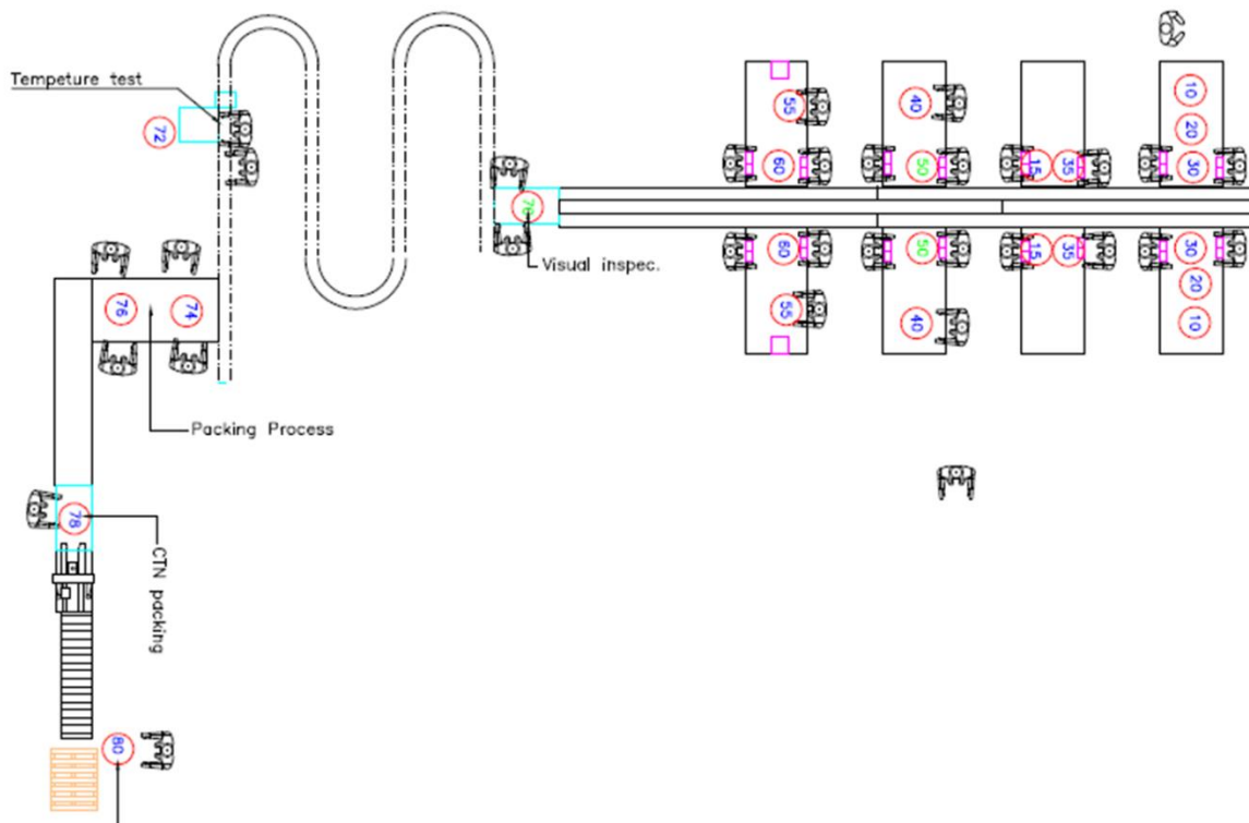
Figura 4-26 Línea de manufactura desacoplada (ASMD, 2017)
